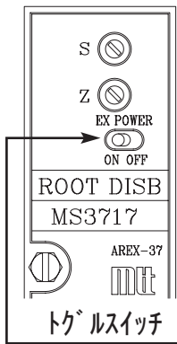
MS3717本体上面
