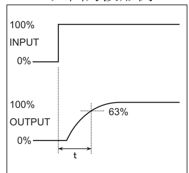
入出力波形例
